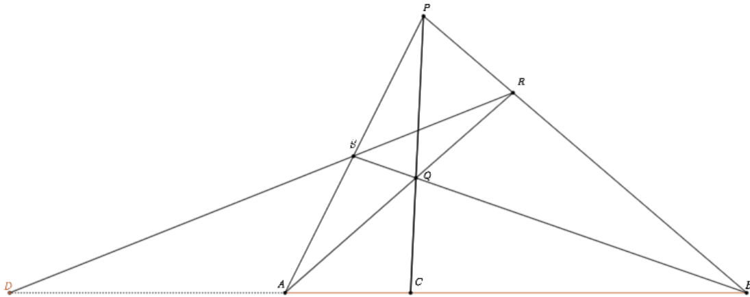
Figura 5. Construção de conjugado harmônico com régua não graduada.
